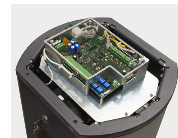
Плата управления
