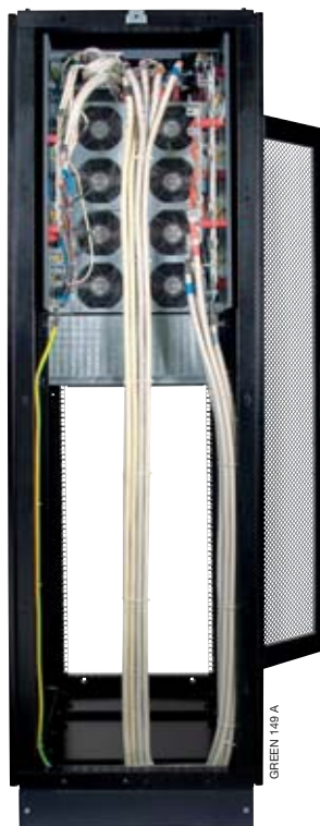
Обзор сзади (до установки задней защитной крышки).
