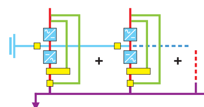
Совместно используемая аккумуляторная батарея
