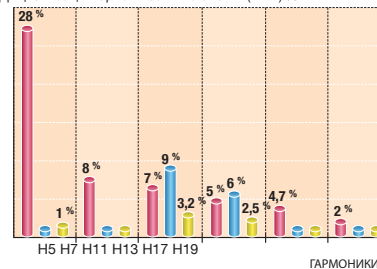
Коэффициент общих гармонических искажений (THDI) %
