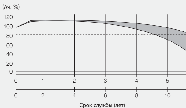
Срок службы свинцовых аккумуляторных батарей при 20 °C
