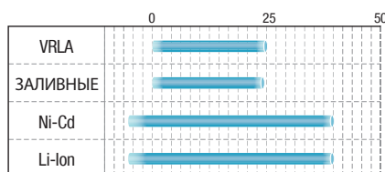
Температура деградации (°C)
